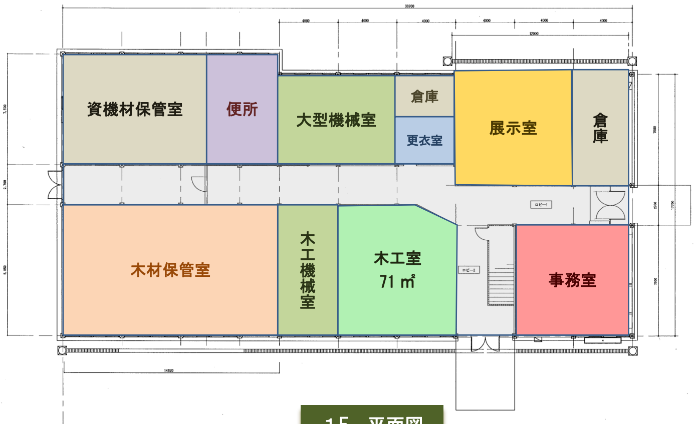
1F 平面図
